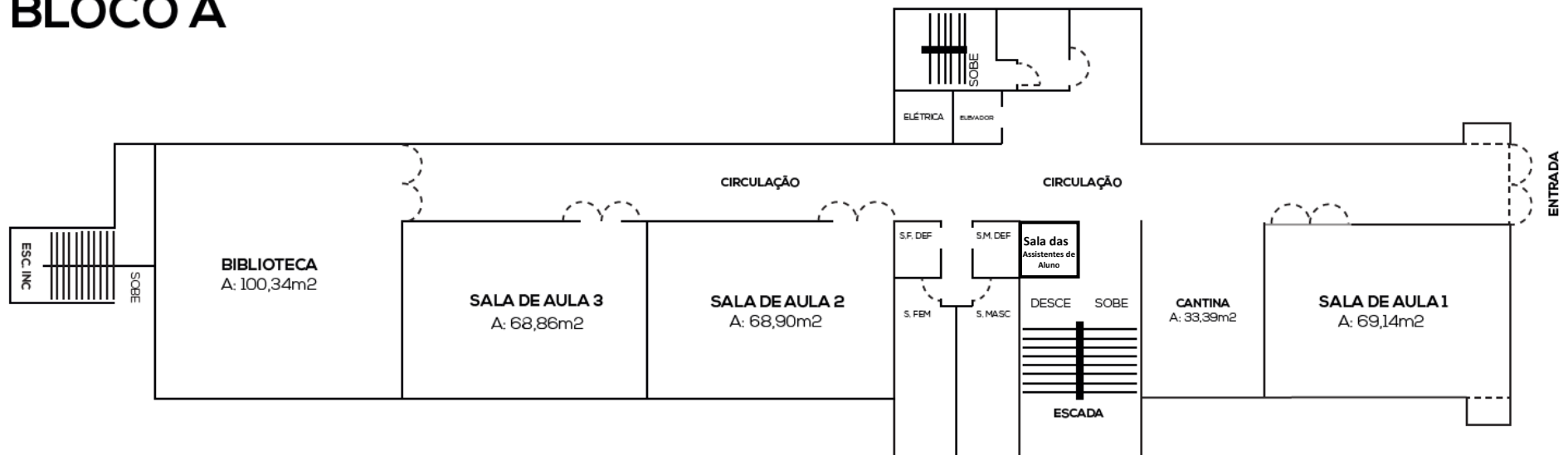
PLANTA TÉRREO - BLOCO A
