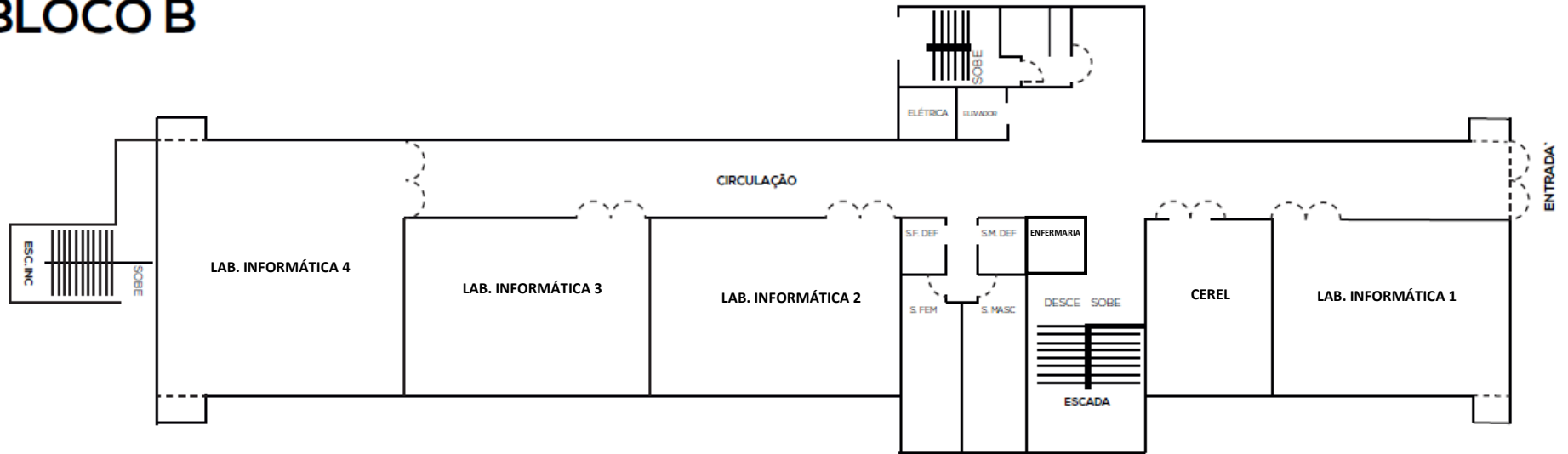
PLANTA TÉRREO - BLOCO B
